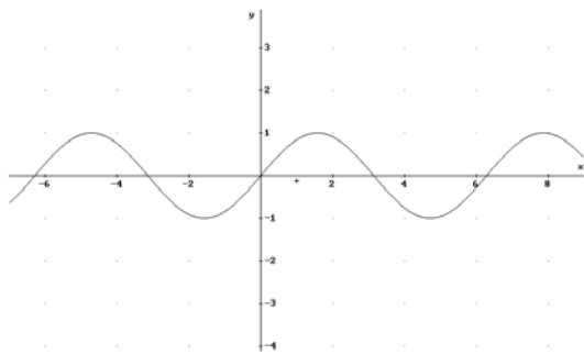
y = \text{sen } x
