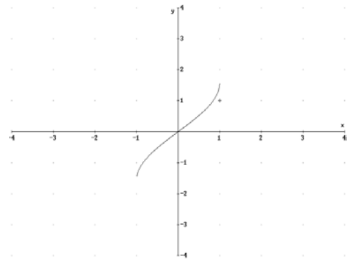
y = \text{arcsen } x
