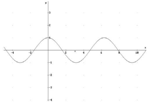
y = \text{cos } x
