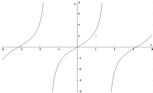
y = \text{tg } x
